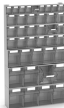
ESTANTERÍA CON 40 CAJONES VISUAL BOX DIM. (mm): A=602 P=190 H=1000
