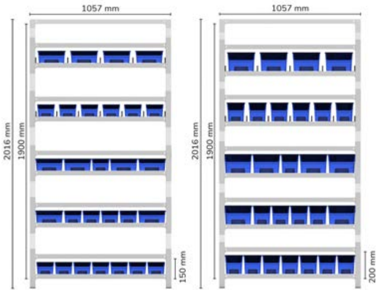
Schéma disposition bacs RK Box Air sur rayonnage ST et armoire à portes battantes Perform
