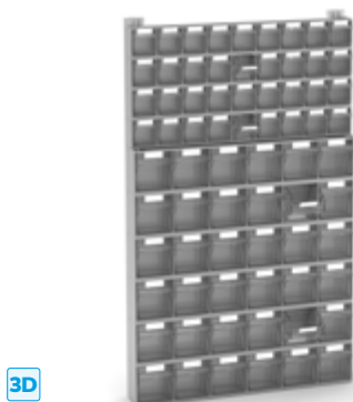
RAYONNAGE AVEC 72 TIROIRS VISUAL BOX DIM. (mm): L=602 P=114 H=1000
