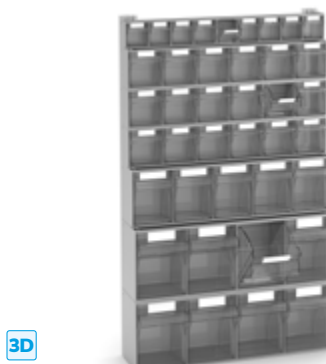
RAYONNAGE AVEC 40 TIROIRS VISUAL BOX DIM. (mm): L=602 P=190 H=1000
