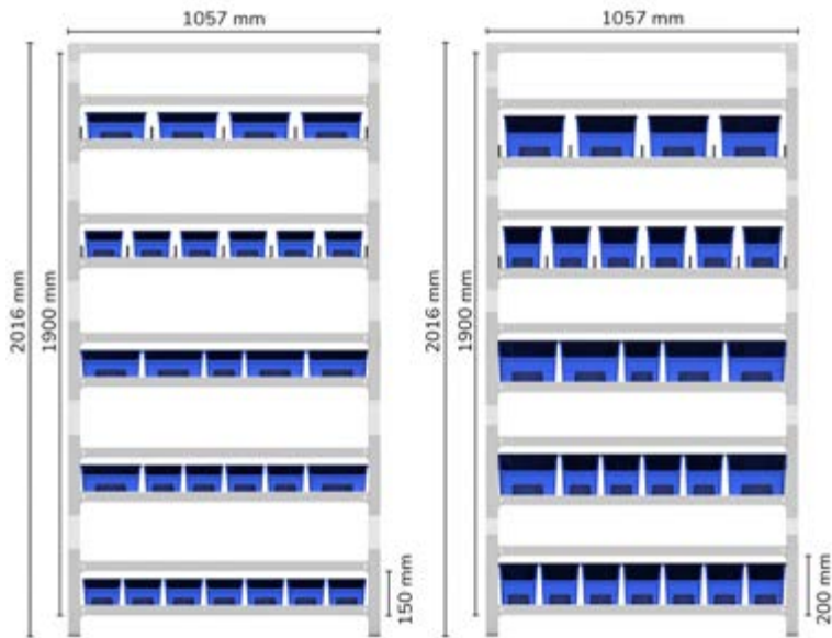
Schema der Anordnung der Kästen RK Box Air auf Regal ST und Schrank mit Flügeltüren Perform
