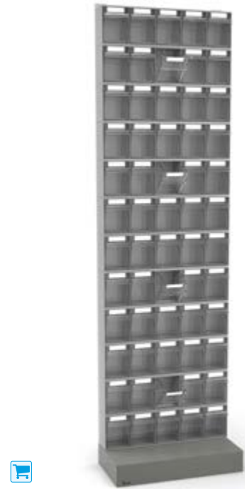
REGALE MIT 60 SCHUBLADEN VISUAL BOX ABM. (mm): B=604 T=322 H=2100
