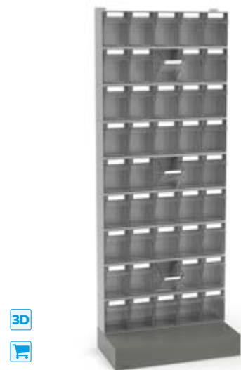
REGALE MIT 45 SCHUBLADEN VISUAL BOX ABM. (mm): B=604 T=322 H=1600
