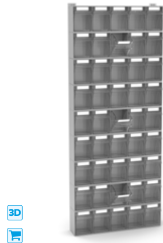
REGALE MIT 45 SCHUBLADEN VISUAL BOX ABM. (mm): B=602 T=157 H=1500
