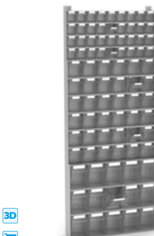
SCAFFALE CON 87 CASSETTI VISUAL BOX DIM. (mm): L=602 P=157 H=1500
