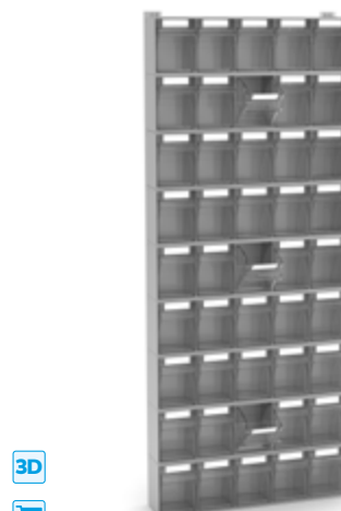
SCAFFALE CON 45 CASSETTI VISUAL BOX DIM. (mm): L=602 P=157 H=1500
