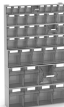
RAYONNAGE AVEC 40 TIROIRS VISUAL BOX DIM. (mm): L=602 P=190 H=1000
