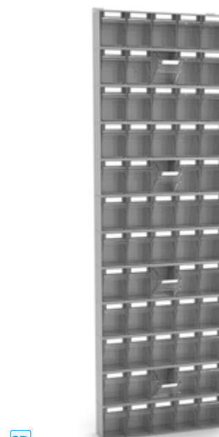
RAYONNAGE AVEC 60 TIROIRS VISUAL BOX DIM. (mm): L=602 P=157 H=2000
