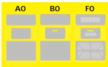
Kästen mit geschlossenem Boden Art. F PB 6851 BO 01 Außenabmessungen: mm 600x400x220h Nutzabmessungen innen: mm 555x355x200h
